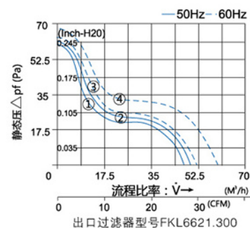
功率特性曲线 FKL 6621....
