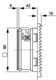
风扇及过滤器 FKL 6621.230
