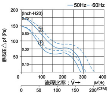
出口过滤器 型号FK8925.300
