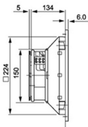
风扇及过滤器 FK 8925.230
