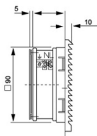
风扇及过滤器 FK 8921.230
