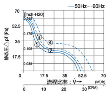
功率特性曲线 FK 8921....
