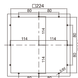
安装剖面 FKS5625-162....
