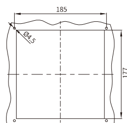
安装剖面 FKL9923-150....
