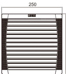
风扇及过滤器 FKL5525-150.230....
