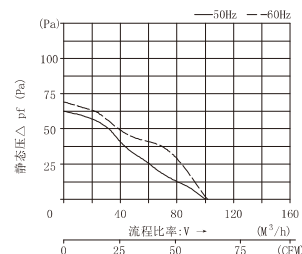
功率特性曲线 FKL6623....
