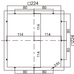
安装剖面 FKL5525-162....
