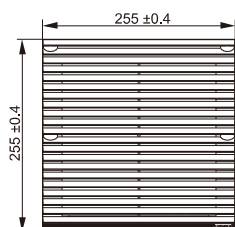
风扇及过滤器 FKL6625.230-D....
