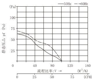
功率特性曲线 FK8923....
