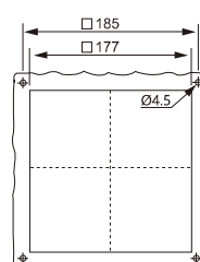
安装剖面 FKL6623....
