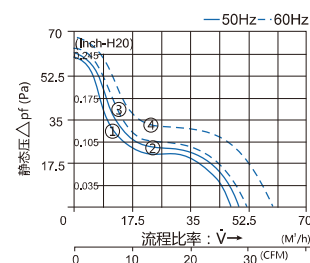
功率特性曲线 FKL6621....
