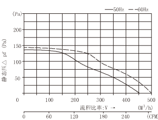
功率特性曲线 FKL6626....
