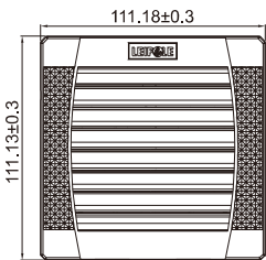
风扇及过滤器 FKL5521.024/230....
