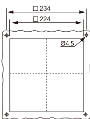
安装剖面 FKL6625....
