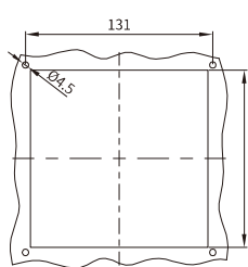
安装剖面 FKL9922....
