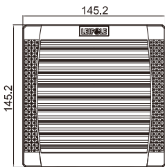
风扇及过滤器 FKL5522.230....
