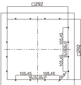
安装剖面 FKL5526-D....
