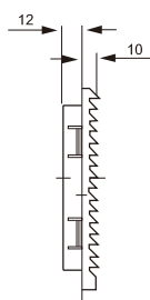
出口过滤器 FKL6621.300
