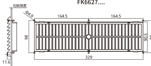
安装剖面 FK6627....
