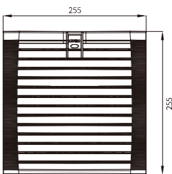
风扇及过滤器 FKL9925.230-D....
