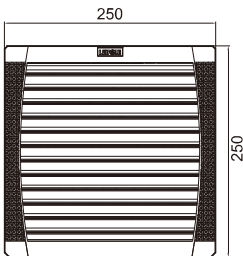
风扇及过滤器 FKL5525-200.230....
