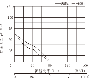
功率特性曲线 FKL6622....
