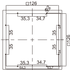
安装剖面 FKL5522....
