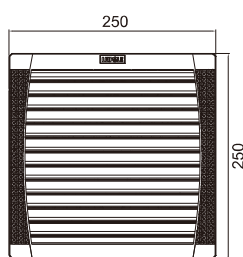
风扇及过滤器 FKL5523.230....
