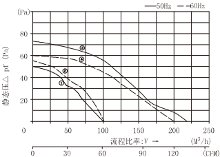
功率特性曲线 FB9804....
