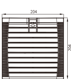
风扇及过滤器 FKL9923-162.230....
