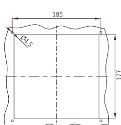
安装剖面 FKL9923-162....
