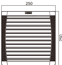
风扇及过滤器 FKL5525-162.230....
