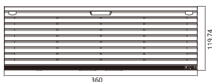
出口过滤器 FK6627.300
