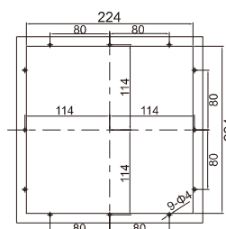
安装剖面 FKL5523....
