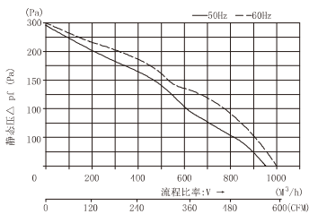
功率特性曲线 FK9926-D....
