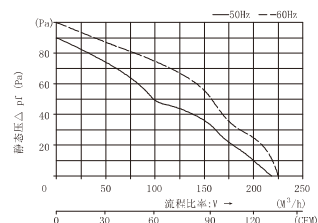
功率特性曲线 FK9925....
