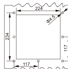
安装剖面 FKL6625....
