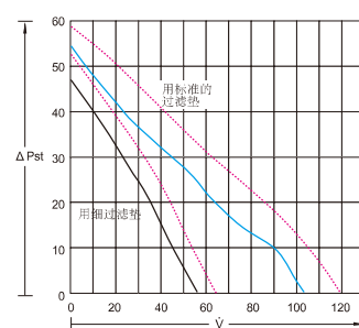
功率特性曲线 FK6627....
